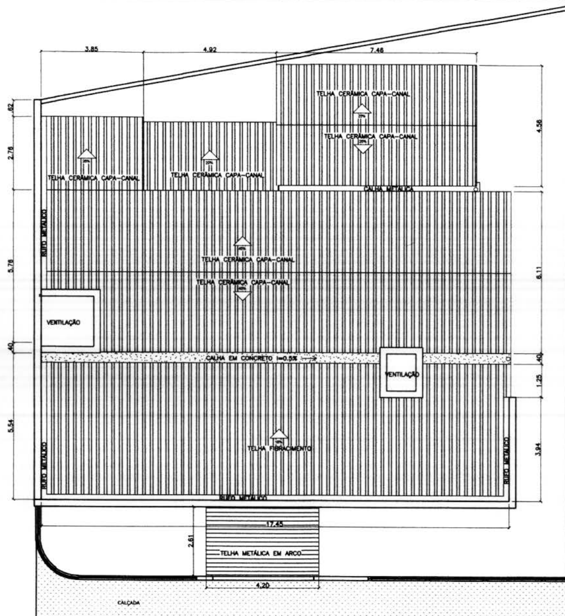
Planta de Cobertura esc 1:100
